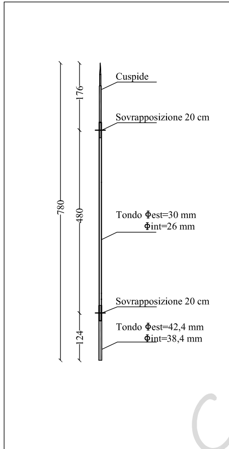
ASTA DI CAPTAZIONE SULLA CROCE
