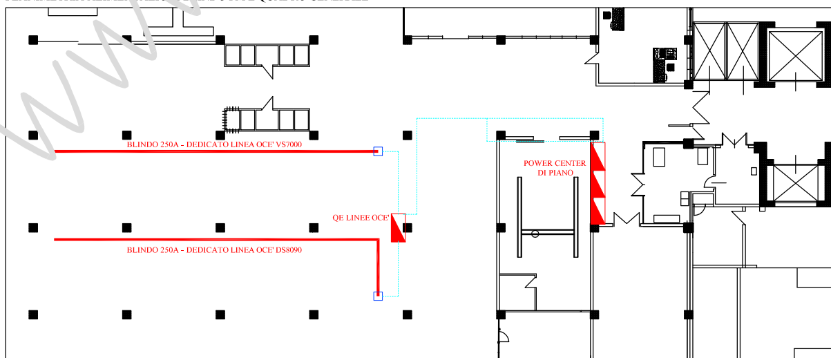
PLANIMETRIA ALIMENTAZIONI BLINDO FM E QUADRO GENERALE
